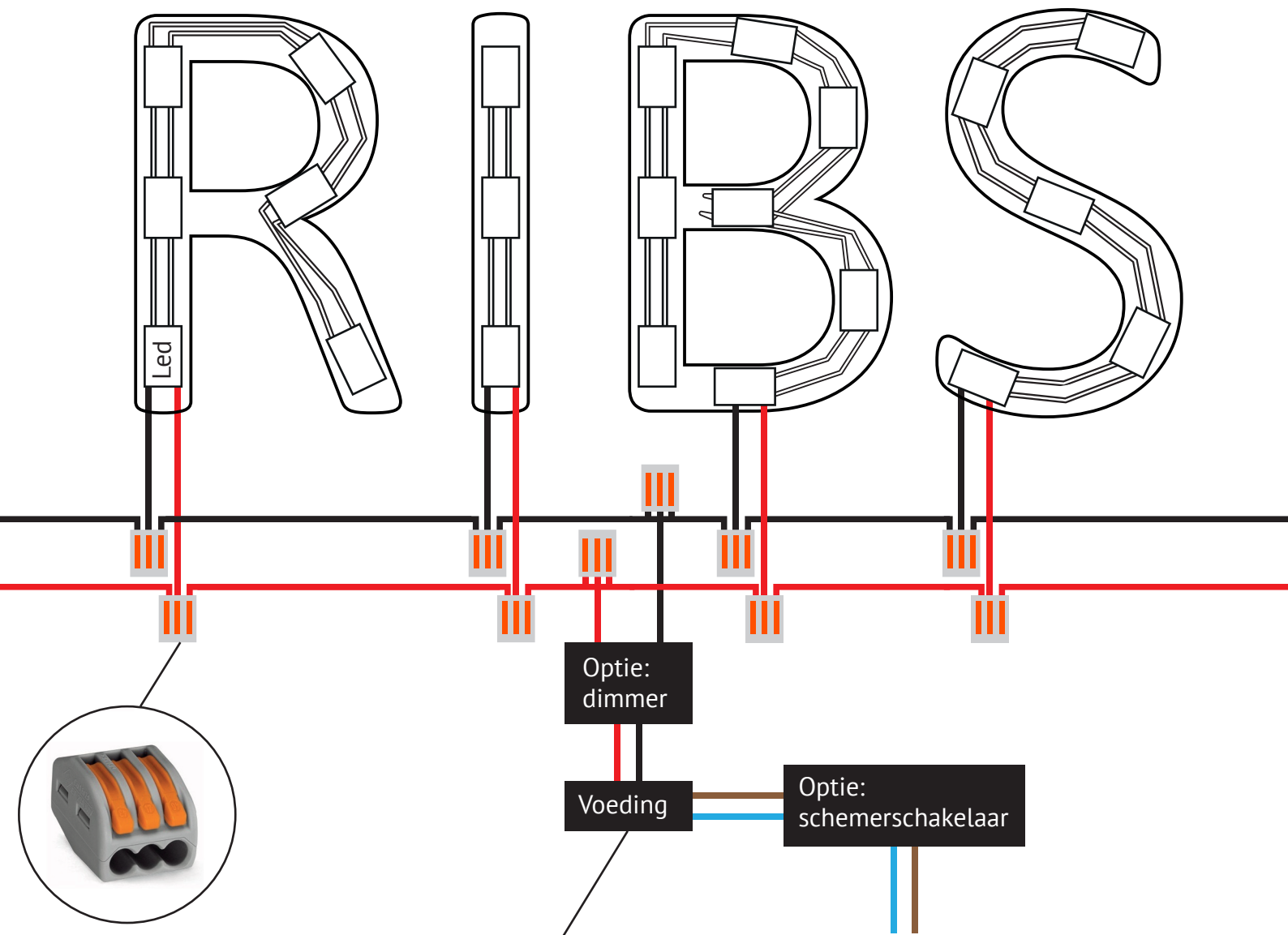
Wago verbindingsklem.
